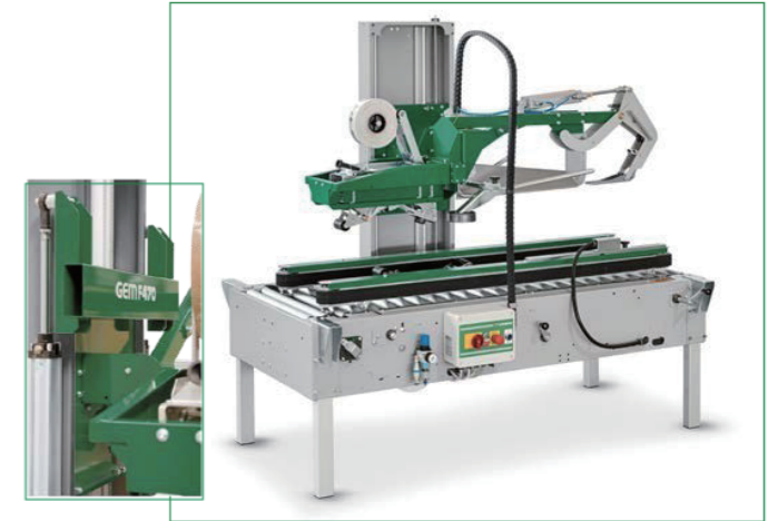
テーピングヘッドの省力昇降装置/GEM-F470G (空圧シリンダータイプ/オプション)
